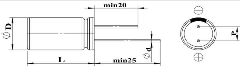
导针型尺寸图示 Dimintions (mm)
